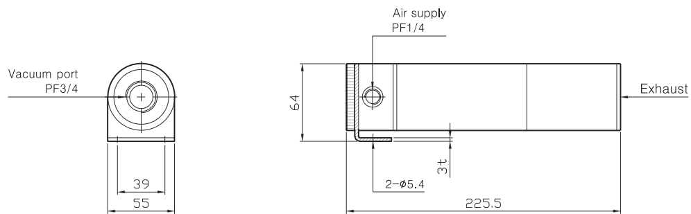
SMR455/655
