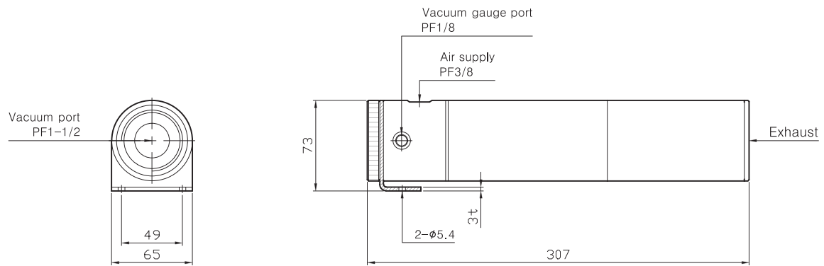
SMR665/865
